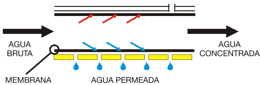
Esquema de filtro Ósmosis reversa.
